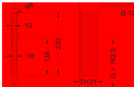
Fräsmaße
