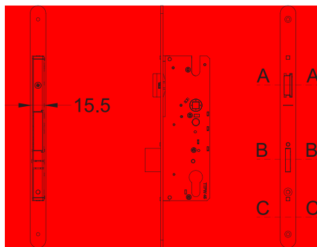
Ansichten
